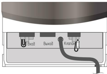
б) с разъемом для кабеля клапана
