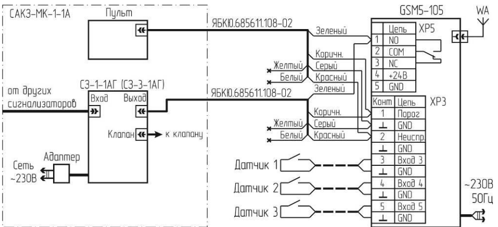
Рисунок Б.4 – Схема подключения GSM5-105.
