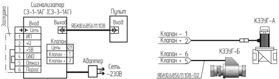
а) сигнализаторы с клеммником «Клапан»
